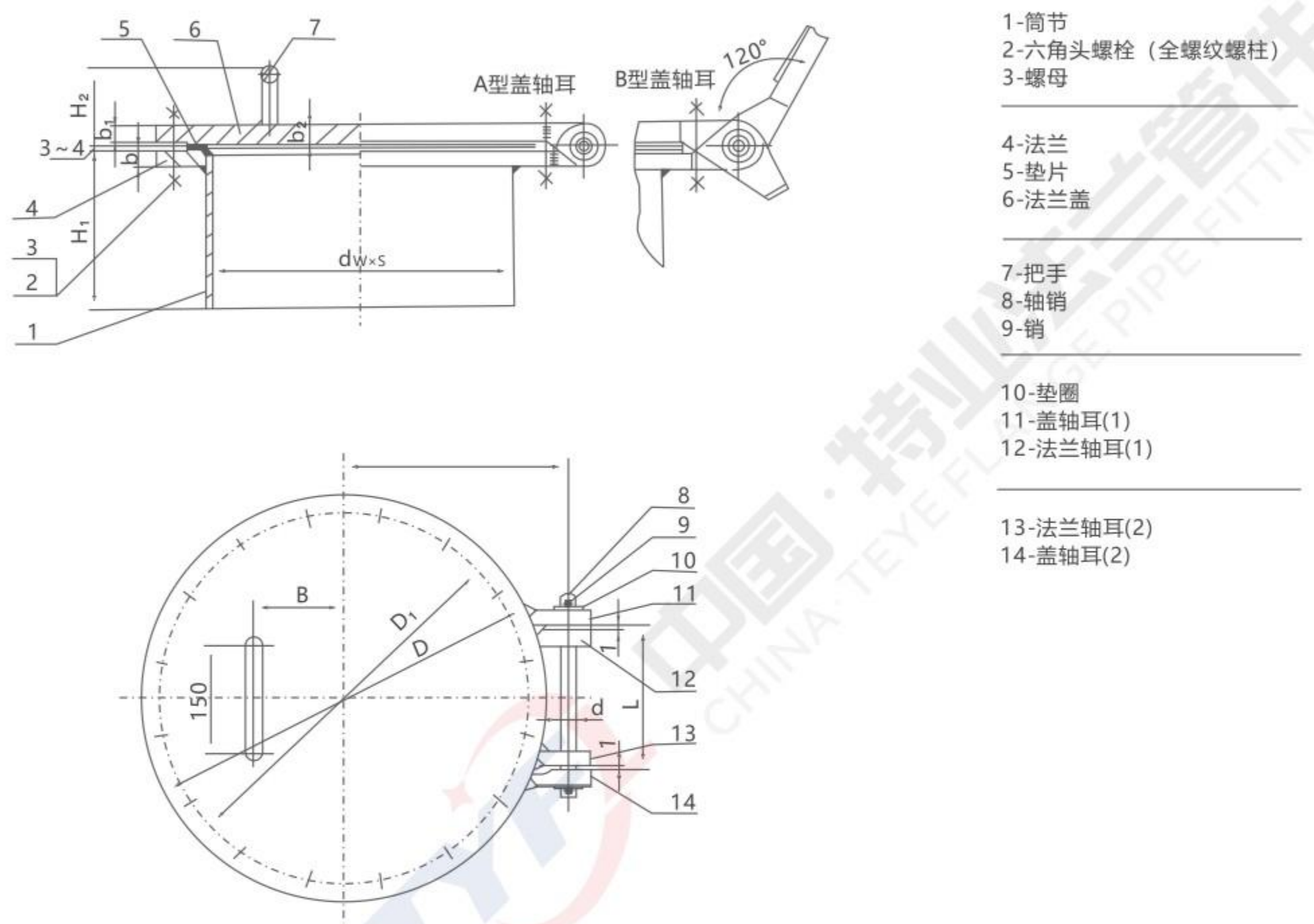
回转盖板式平焊法兰人孔的形式尺寸
