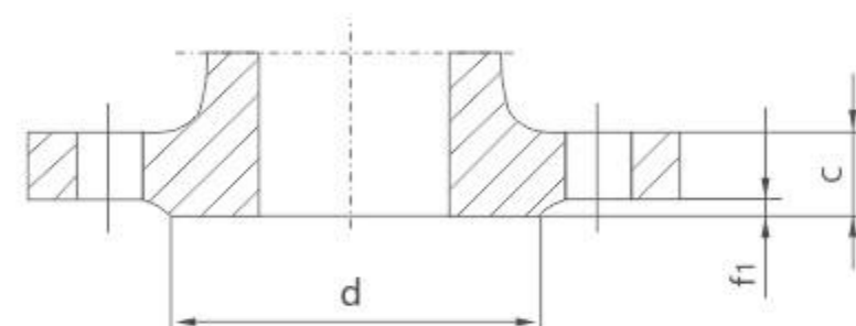
突面 (RF)
