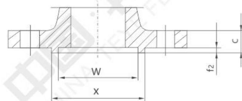
榫面 (T)
