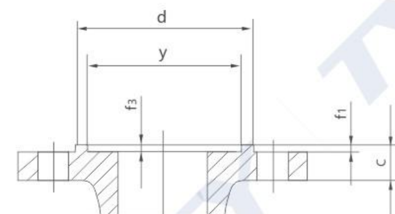
凹面 (FM)
