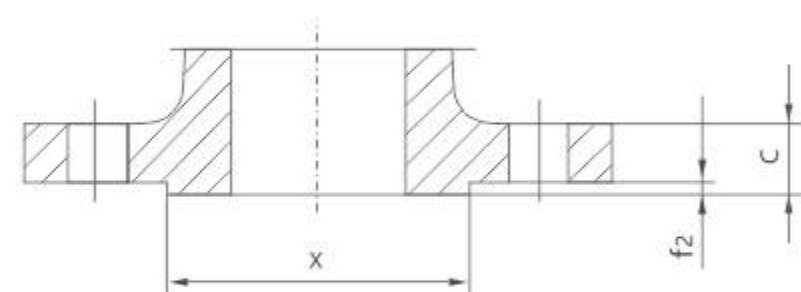
凸面 (M)
