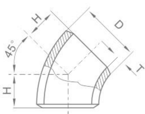
45° 弯头 Elbow
