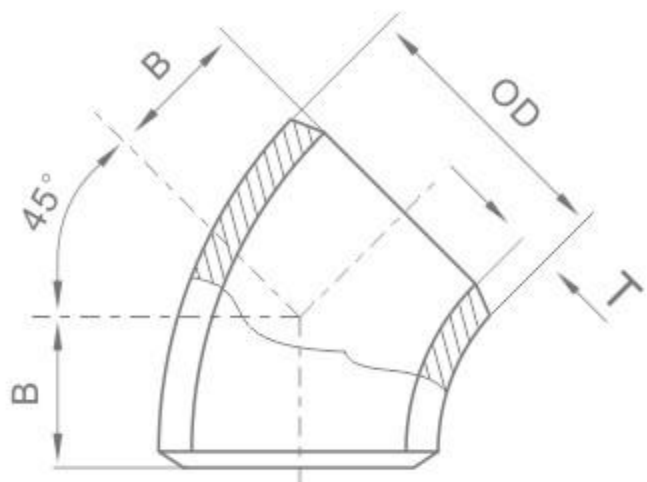
45° 弯头 Elbow
