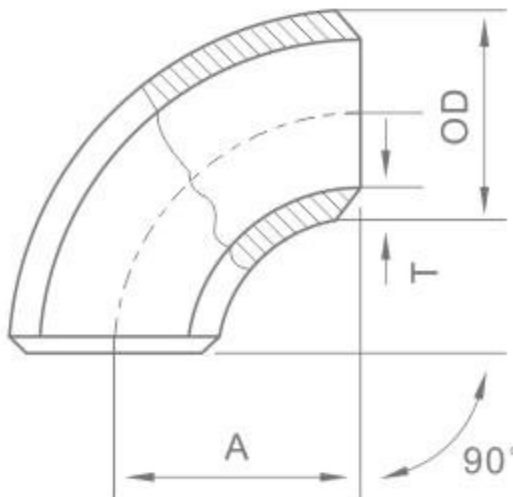
90° 弯头 Elbow
