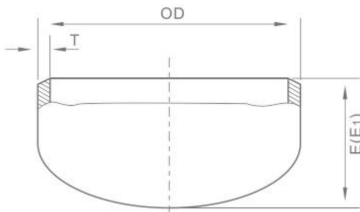
管帽 Cap
