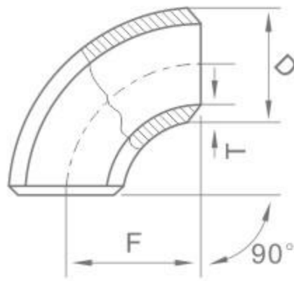
90° 弯头 Elbow
