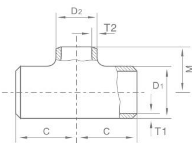
异径三通 Reducing Outlet Tee
