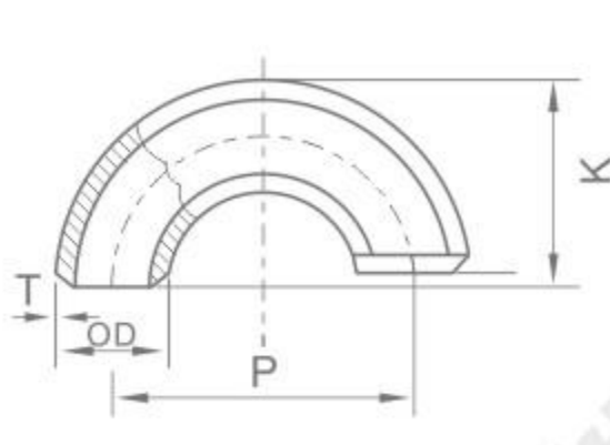
180° 弯头 Elbow
