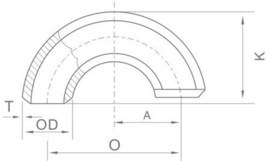
180° 弯头 Elbow
