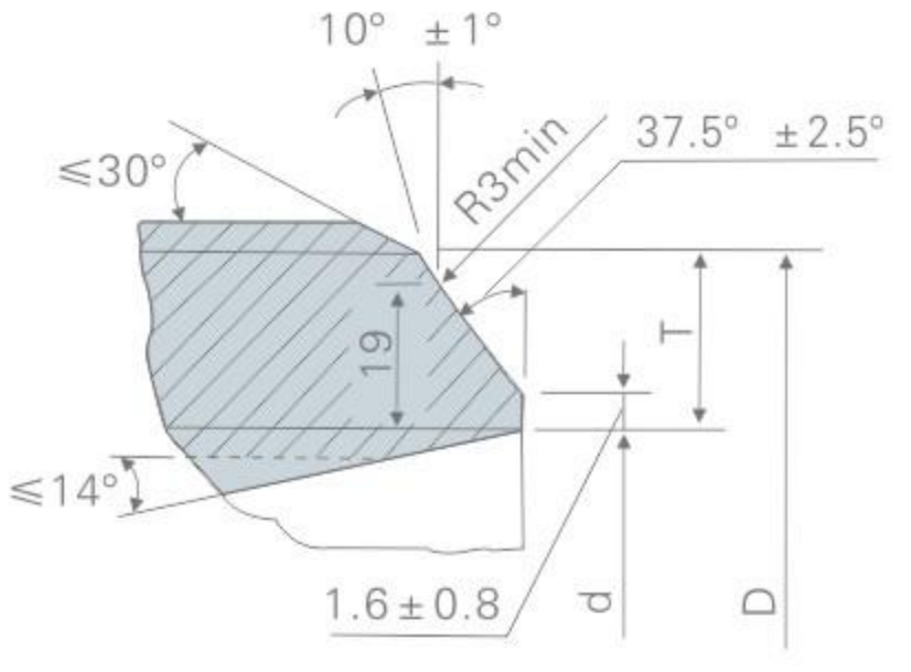
(b) 壁厚 ≥ 22
