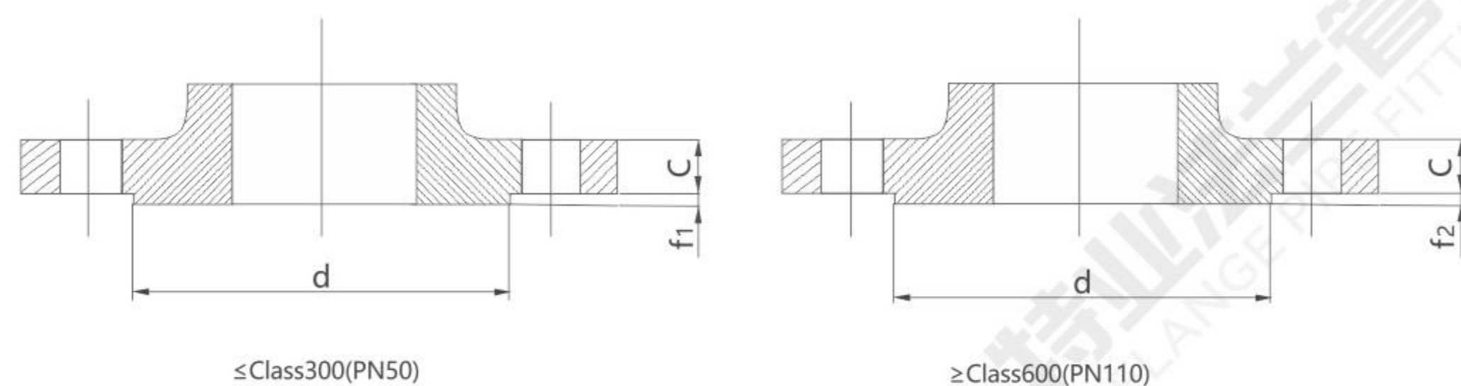
突面法兰 (RF) 面的密封面尺寸
